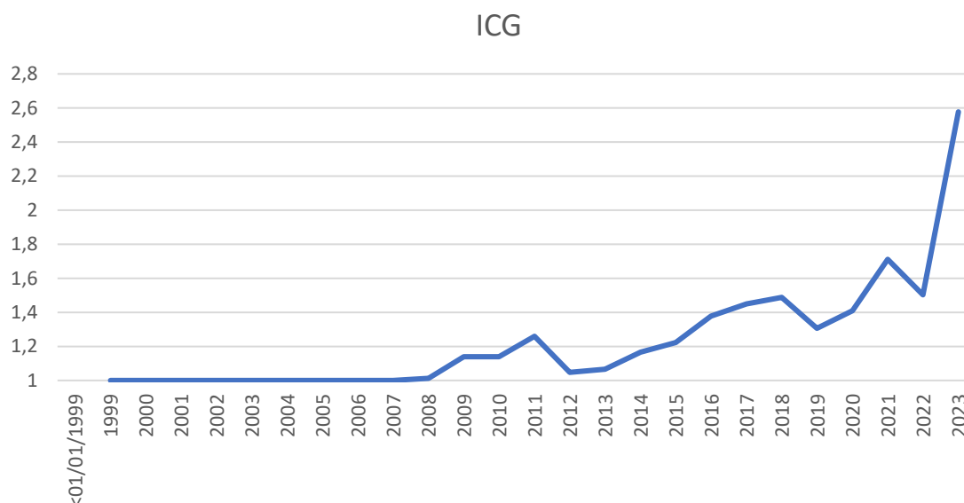
Figura 2. Evolución del coeficiente de conservación genética promedio.
